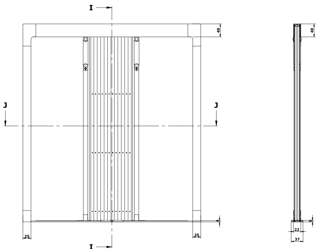
ÚSEK I-I
