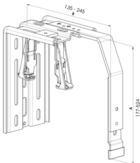
KBT5/1 (B=135-190; A=177-524) KBT5/2 (B=191-245; A=177-524) (pro horní profil 56 x 58)
