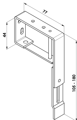
KBT1 (pro horní profil 40 x 40)
