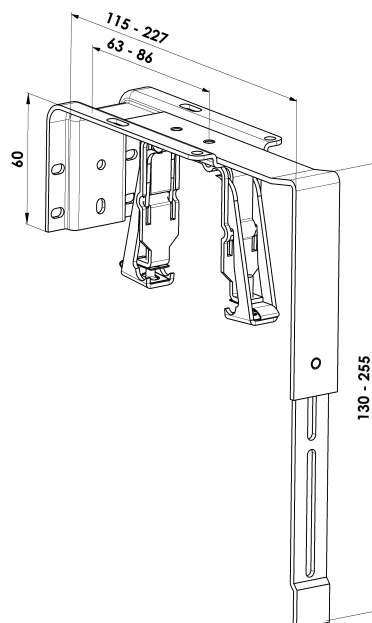
KBT2 (pro horní profil 56 x 58)
