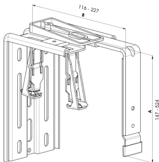
KBT4/1 (B=116-169; A=147-524) KBT4/2 (B=170-227; A=147-524) (pro horní profil 56 x 58)
