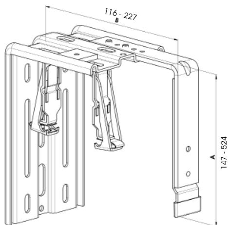
KBT3/1 (B=116-169; A=147-524) KBT3/2 (B=170-227; A=147-524) (pro horní profil 56 x 58)
