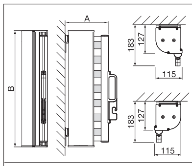
Montáž na stěnu-/Montáž do stropu
