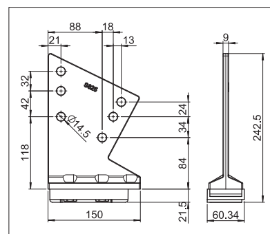
Krokvová konzole
