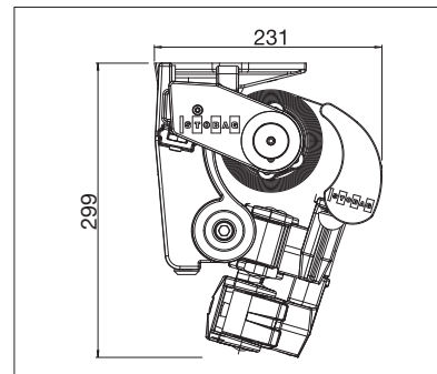
S8133 Montáž do stropu
