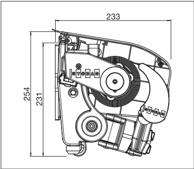
S8135 Montáž na stěnu
