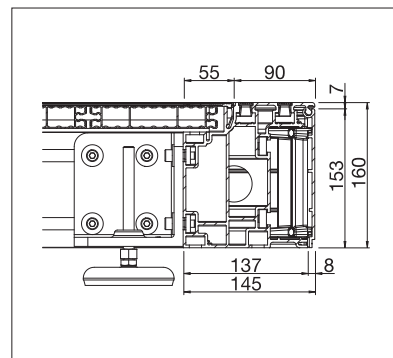
Nastavitelná stojina
