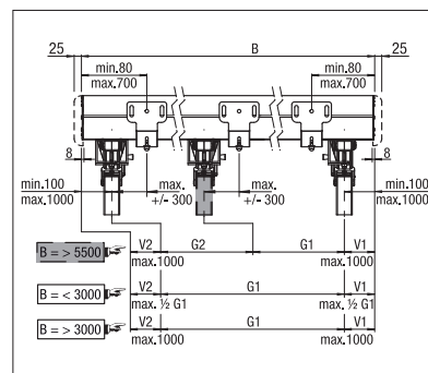
Se třemi vodícími lištami
