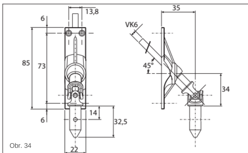
tyčová spojka
