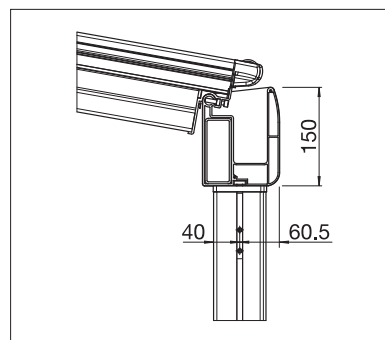
GP5100 | GP5110 Integrovaný okap v příčném nosníku
