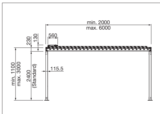
TP6500 Boční pohled
