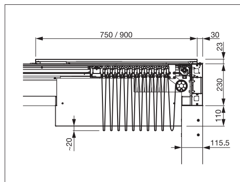
TP6100 Boční pohled (detail vedení potahu)
