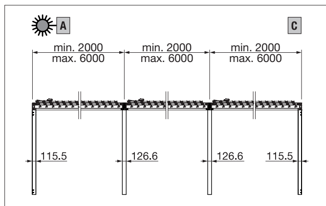
TP6600 - postranní pohled na propojená zařízení
